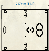
顶视图
